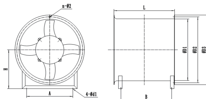
AXF型轴流风机安装尺寸表(直边)管道
