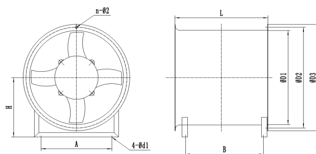
AXF型轴流风机安装尺寸表(喇叭口)管道
